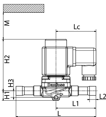
Figure: EVR and DIN plug coil
