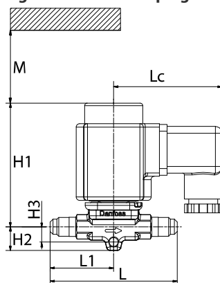
Figure: EVR and DIN plug coil
